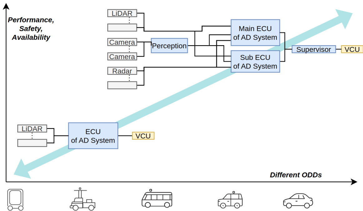
図5 ECU構成例
